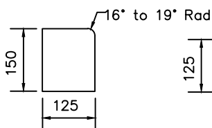
Type BN Fig NA.1a
